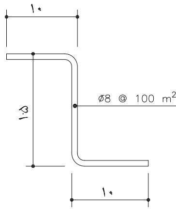
جزئیات بست اتصال
