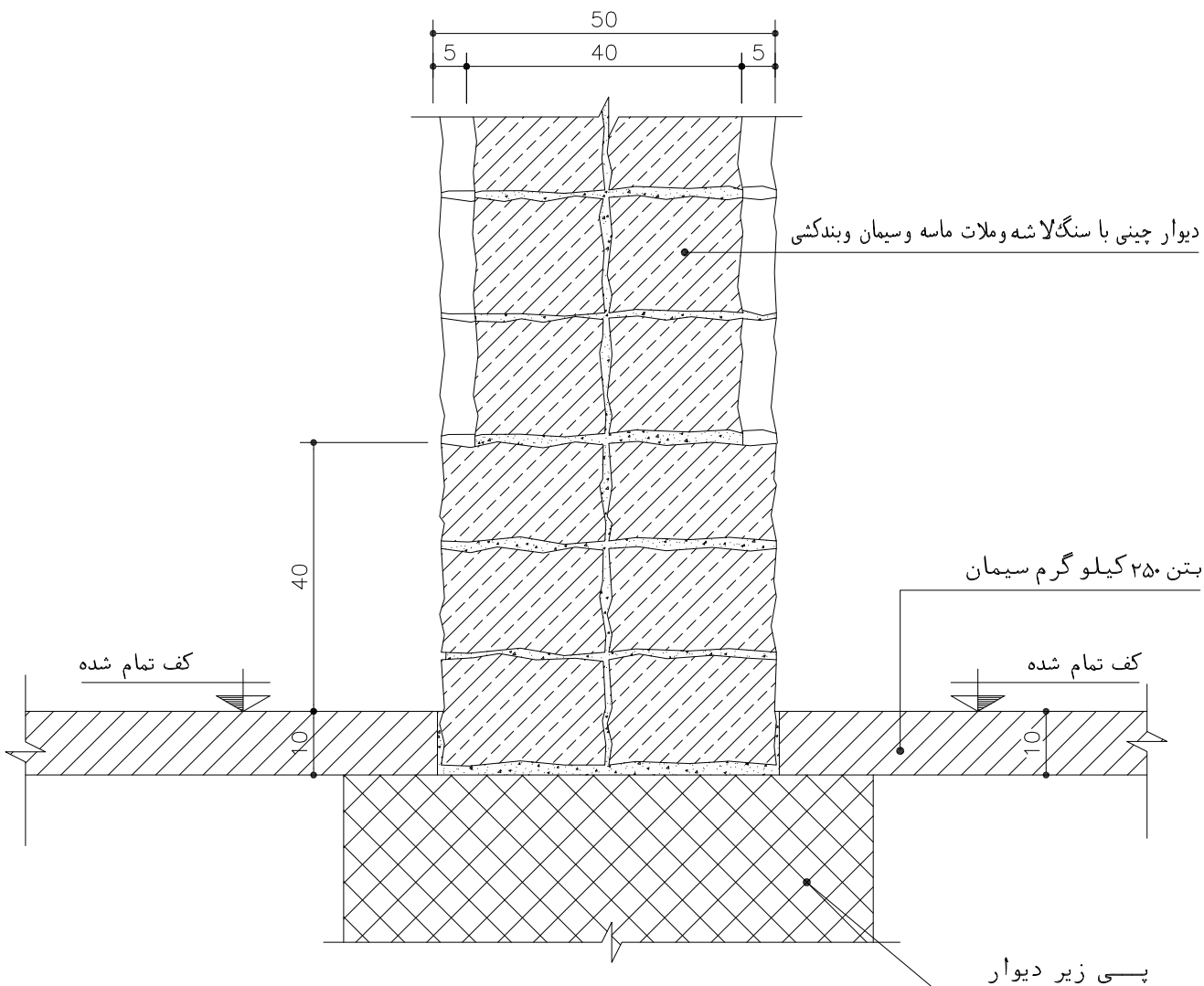
برش (الف - الف)
