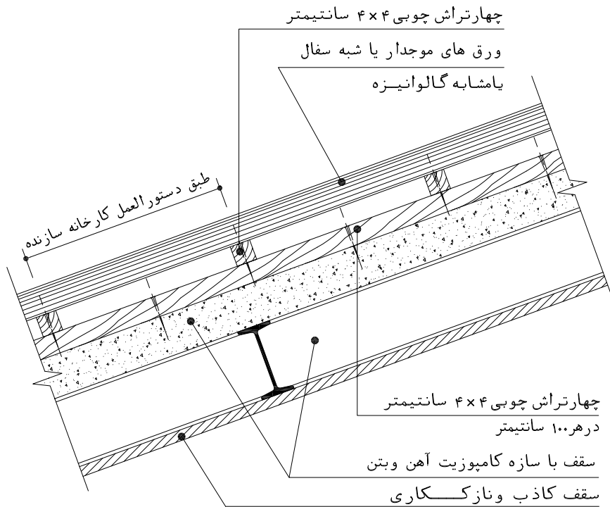
برش سقف در جهت شیب سقف
