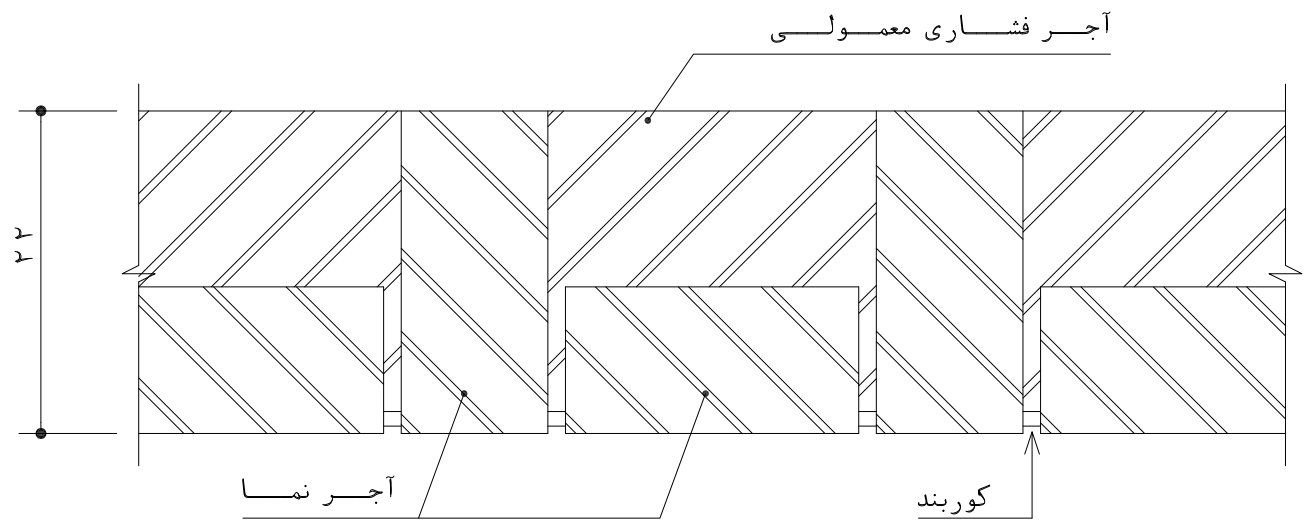
پلان دیوار آجرنمای سنتی با کوربند و بندکشی توگود مقیاس ۱:۵
