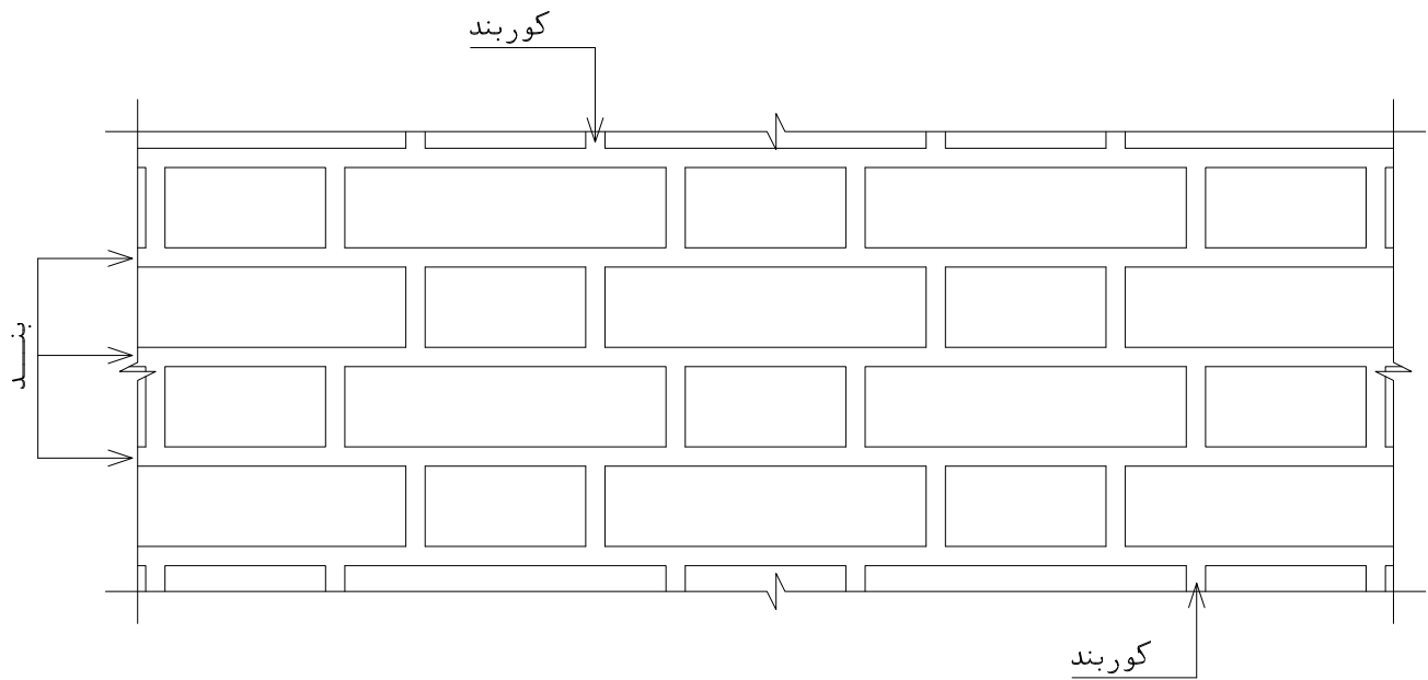
نمای دیوار آجرنمای سنتی با کوربند مقیاس ۱:۵
