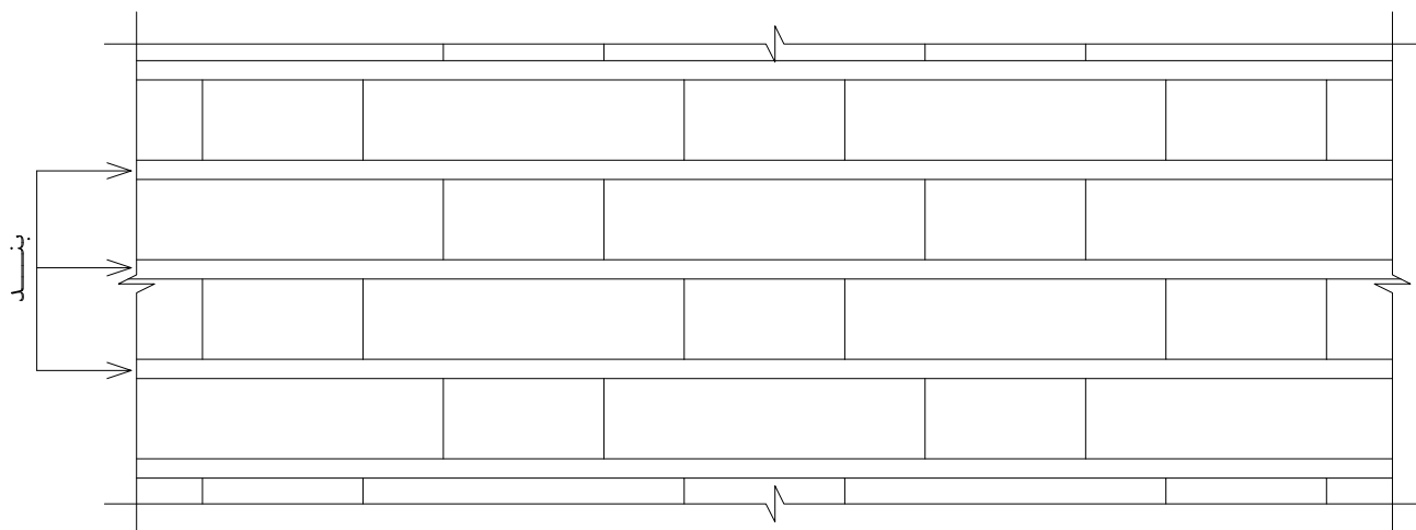
نمای دیوار آجرنمای سنتی بدون کوربند مقیاس ۰.۱:۵
