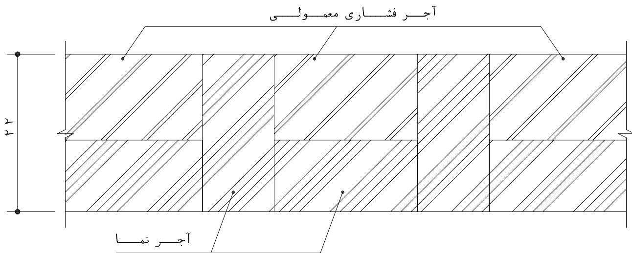
پلان دیوار آجرنمای سنتی بدون کوربند مقیاس ۰.۱:۵
