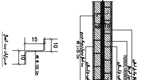
جزئیات دیوار در مجرای در و پنجره
