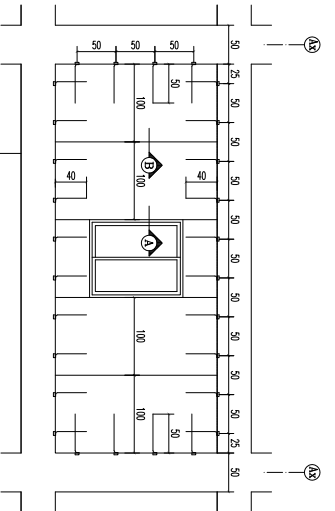
نمای افقی پللی 1/10
